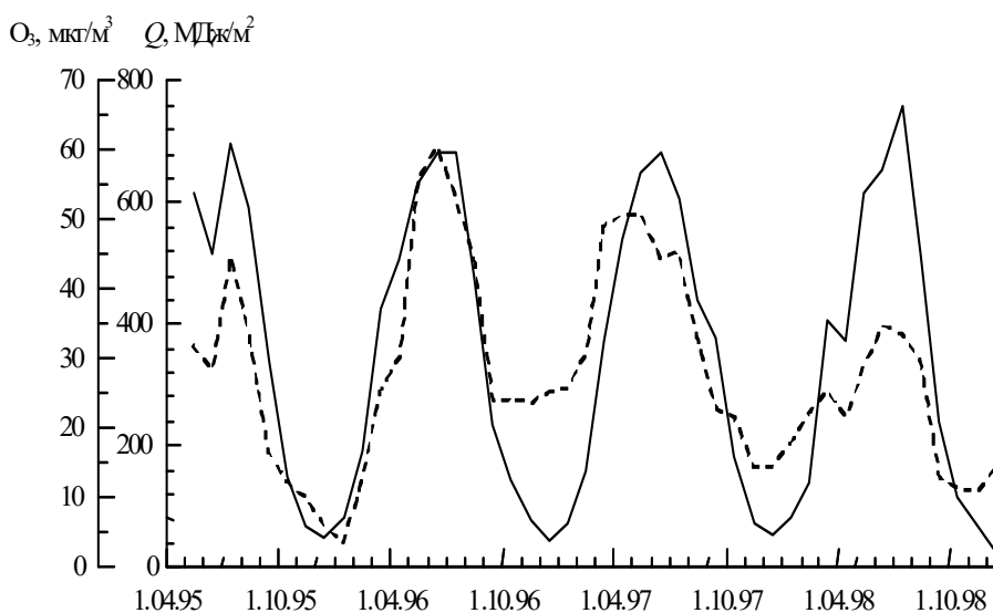
Рис. 2. Многолетний ход суммарной солнечной радиации и концентрации озона в Томске в 1995–1998 гг.: — - суммарная радиация; - - - - озон
