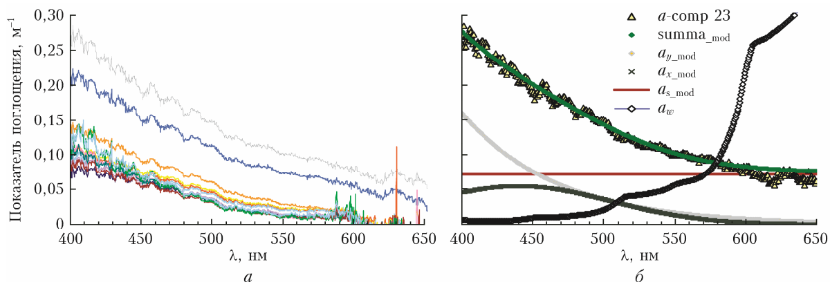
Рис. 5. Спектры суммарного поглощения трех основных природных компонентов морской воды по данным комплекса ЭММА 4.09.2019 г. (а); пример оценки концентрации основных природных компонентов морской воды в единицах поглощения (б): пигментов фитопланктона ( a_x ) на длине волны голубого максимума их поглощения ( a_{x,440} = 0,055 \text{ м}^{-1} ), растворенного органического вещества a_y на \lambda = 500 \text{ нм} ( a_{y,500} = 0,036 \text{ м}^{-1} ) и минеральной взвеси a_s , поглощение которой считается неселективным в этом диапазоне ( a_s = 0,072 \text{ м}^{-1} ) (см. цветной рисунок на сайте http://iao.ru/ru/content/vol.36-2023/iss.12 )
