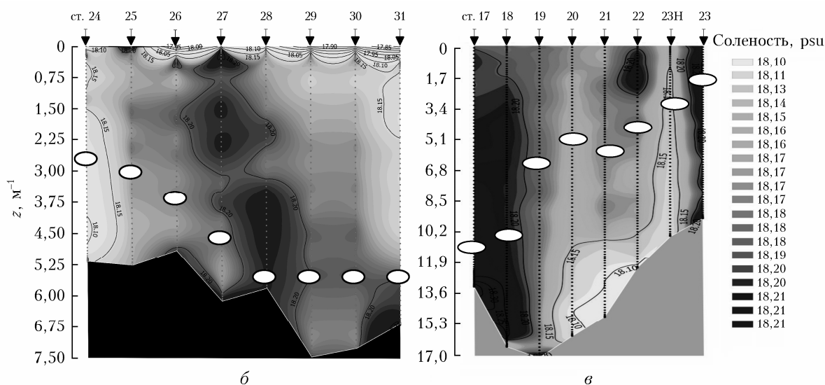
Рис. 6. Сопоставление результатов, полученных с помощью комплекса ЭММА, и проб воды с поверхности после фильтрации (а); сравнение с картиной распределения солености по глубине 3 (б) и 4 сентября 2019 г. (в); овалы — глубина видимости диска Секки
