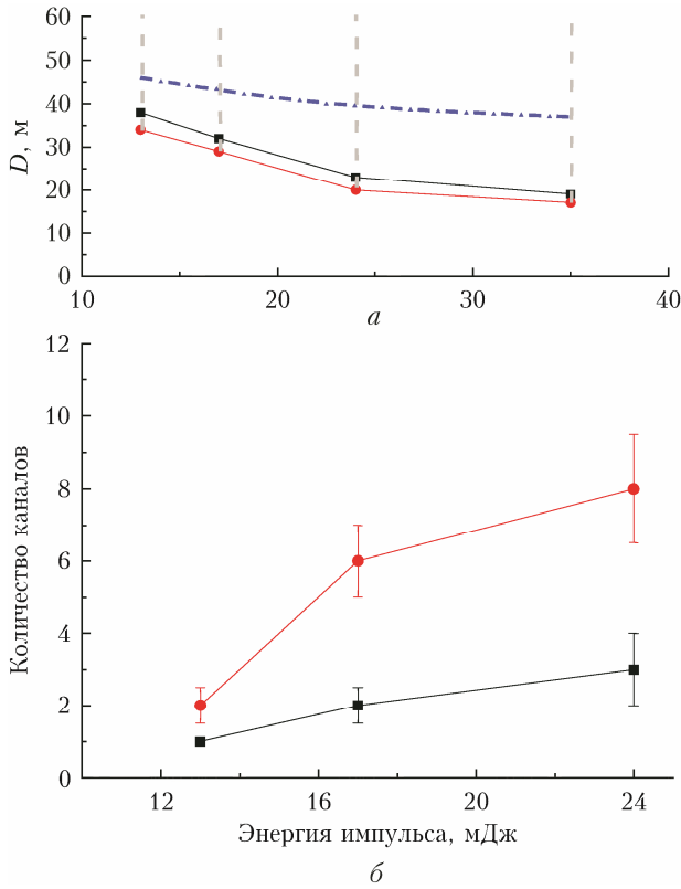
Рис. 3. Зависимость начала (сплошные кривые) и конца ОМФ (штрихпунктирная кривая) ( a ) и количества каналов ( b ) от энергии фемтосекундного лазерного импульса при наличии (—●—) и отсутствии турбулентности (—■—) для пучка с d = 2,5 см; штриховые прямые – интенсивные световые каналы
