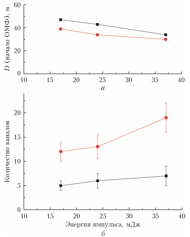
Рис. 4. Зависимость начала ОМФ ( a ) и количества каналов ( b ) от энергии фемтосекундного лазерного импульса при наличии (—●—) и отсутствии турбулентности (—■—) для пучка диаметром 5 см
