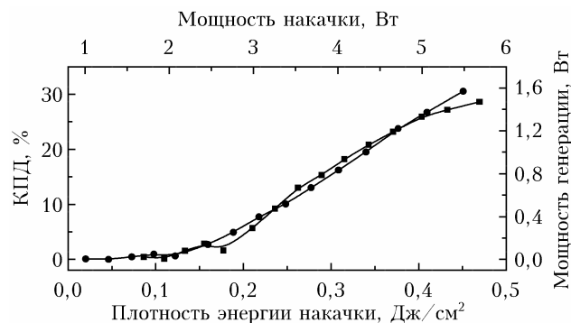
Рис. 14. Зависимость КПД генерации излучения от плотности энергии накачки (■); зависимость средней мощности генерируемого излучения от мощности излучения накачки (●)
