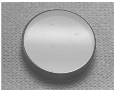
Рис. 7. Диэлектрическое зеркальное покрытие, нанесенное на подложку из ZnSe
