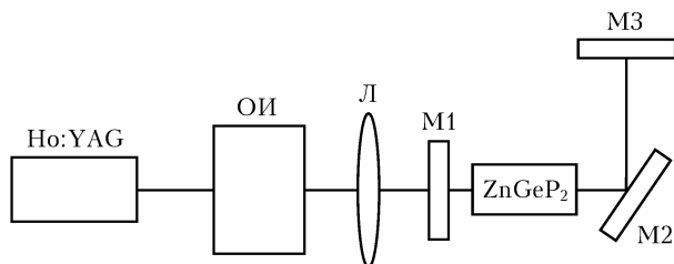
Рис. 13. Схема ПГС на базе монокристалла \text{ZnGeP}_2 с оптической накачкой \text{Ho:YAG} -лазером: ОИ — оптический изолятор; Л — линза; М1 — входное зеркало резонатора; М2 — изготовленное поворотное зеркало; М3 — глухое зеркало резонатора
