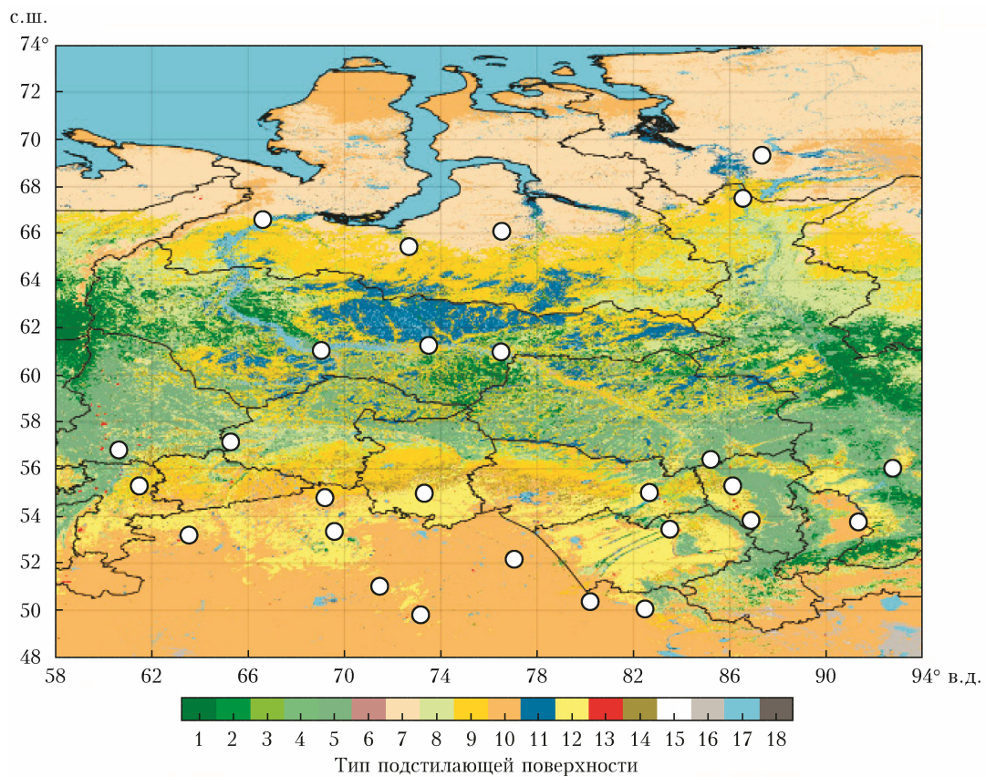
Рис. 1. Расположение АМСГ (белые круги) в Западной Сибири с учетом типа подстилающей поверхности (цветовая шкала): 1 – вечнозеленые хвойные леса; 2 – вечнозеленые лиственные леса; 3 – листопадные хвойные леса; 4 – листопадные лиственные леса; 5 – смешанные леса; 6 – сомкнутые заросли кустарников; 7 – открытые заросли кустарников; 8 – лесостепи; 9 – степи; 10 – луга; 11 – постоянные водно-болотные угодья; 12 – возделываемые земли; 13 – городские и застроенные земли; 14 – естественная растительность; 15 – постоянный снег и лед; 16 – бесплодные земли; 17 – водоемы; 18 – неклассифицированные
