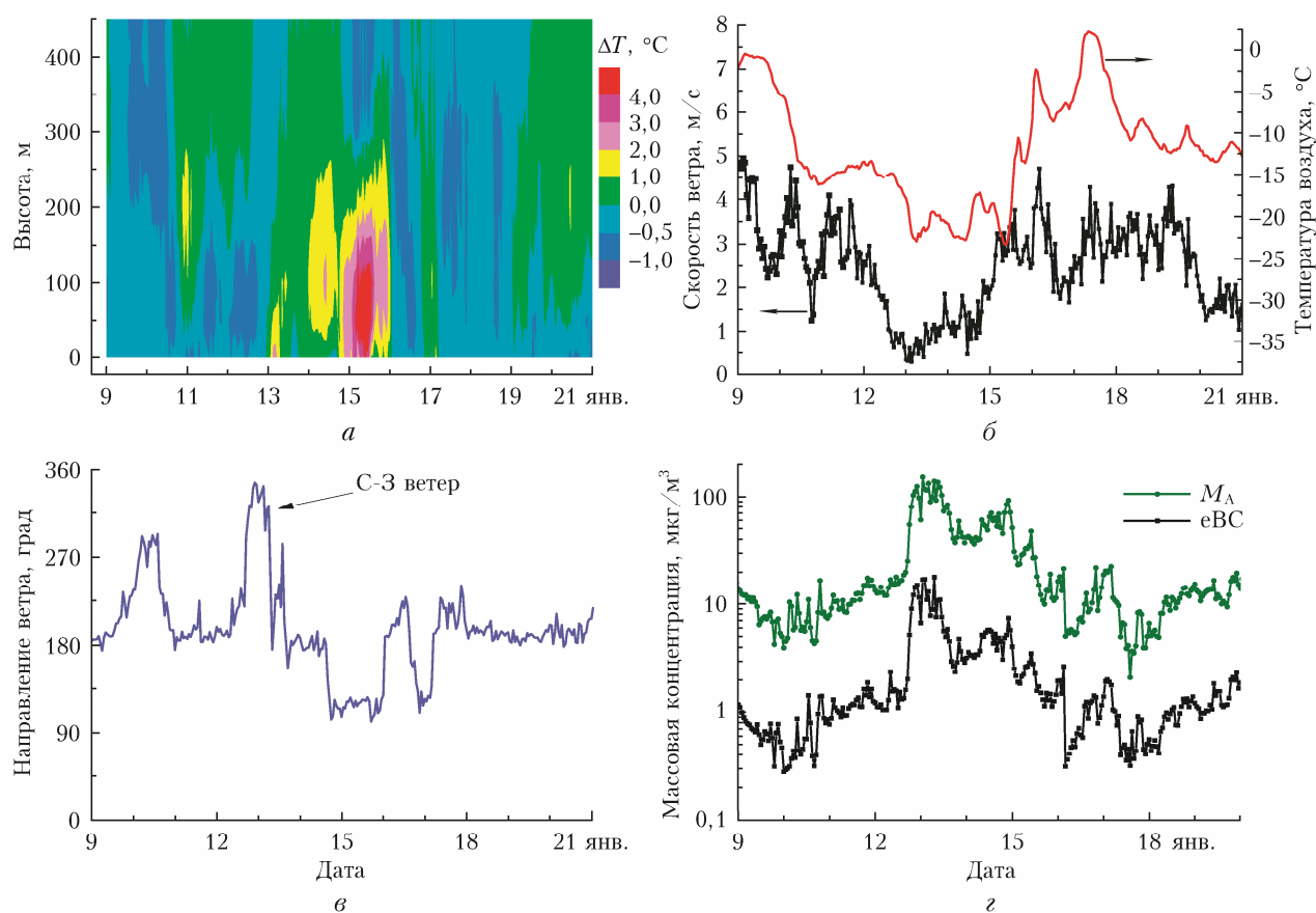
Рис. 3. Метеоситуация и аэрозольные концентрации 12–14 января 2022 г.: а – высотное-временное распределение разности температур; б – скорость ветра, приземная температура; в – направление ветра; г – массовые концентрации субмикронного аэрозоля и черного углерода
