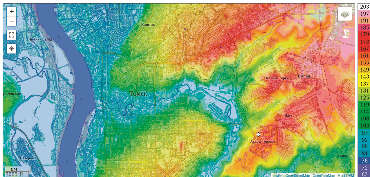
Рис. 2. Фрагмент карты Томска с рельефом местности; ромбом отмечено местоположение Аэрозольной станции и температурно-ветрового комплекса ИОА СО РАН
