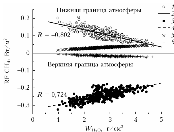
Рис. 2. Радиационный форсинг \text{CH}_4 на нижней (1) и верхней (3) границах атмосферы; 2, 4 – линейная регрессия; 5, 6 – вклад континуального поглощения \text{H}_2\text{O} в \text{RF CH}_4 при различном влагосодержании W_{\text{H}_2\text{O}} в атмосфере
