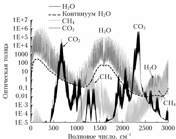
Рис. 1. Атмосферные оптические толщ парниковых газов и континуального поглощения водяного пара на вертикальной трассе для лета средних широт
