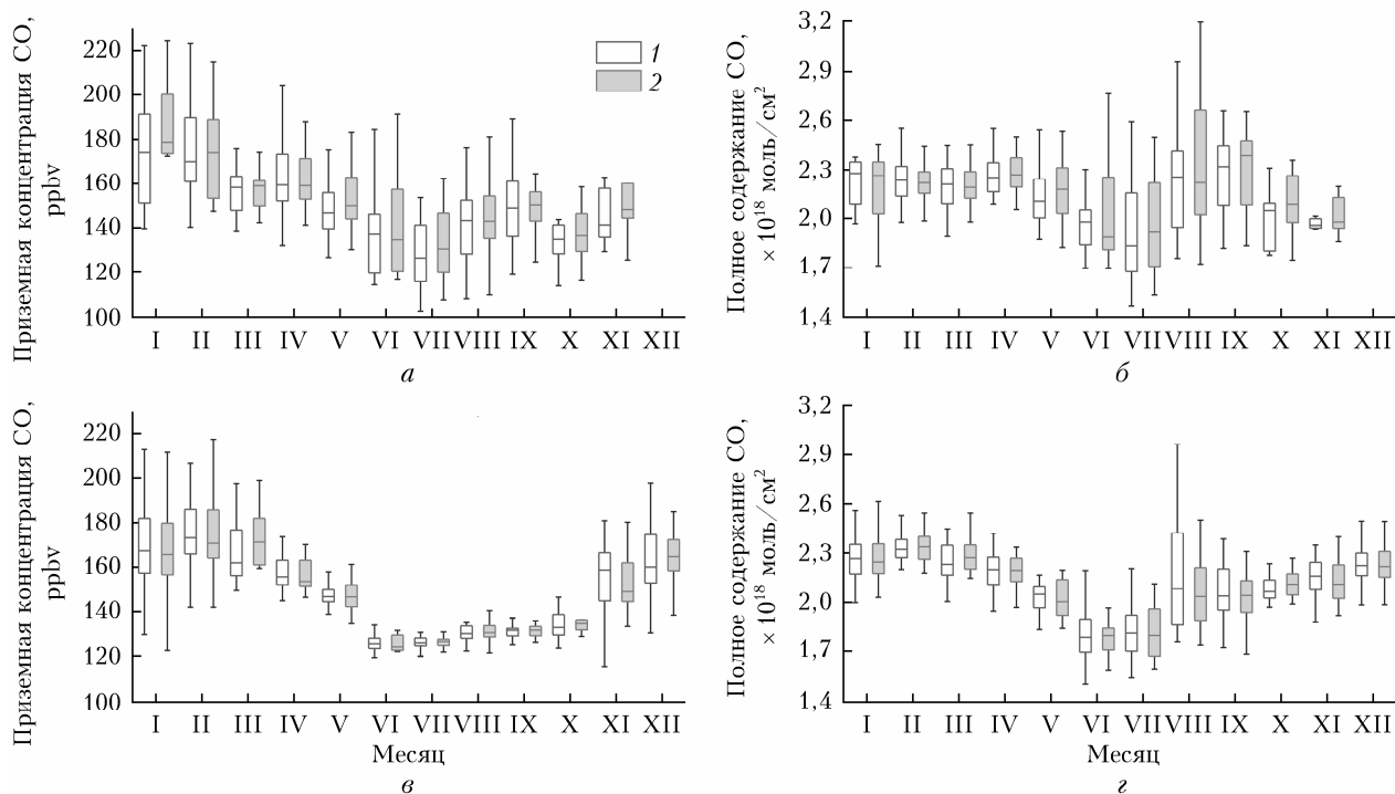
Рис. 4. Диаграммы изменчивости приземной концентрации ( а, е ) и полного (интегрального) содержания СО в тропосфере ( б, з ) в фоновом ( 1 ) и загрязненном ( 2 ) районах для отдельных месяцев по данным МОРИТТ, полученным во время дневных ( а, б ) и ночных ( е, з ) пролетов спутника Тегга за 2020–2023 гг. Дневные данные МОРИТТ в декабре отсутствуют
