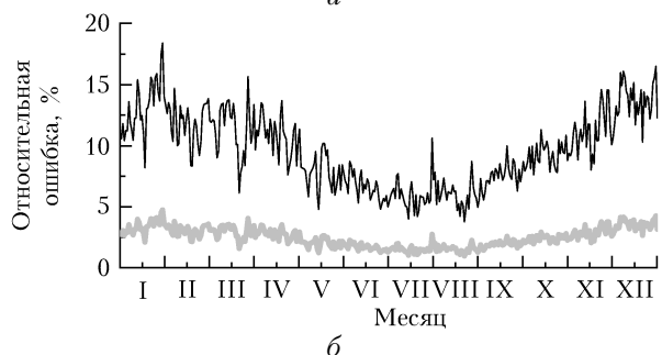
Рис. 2. Средний годовой ход за 1994–2017 гг. со стандартными отклонениями (черные отрезки и кривая), этот же ряд после линейного сглаживания по 15 точкам со стандартными отклонениями (серая кривая) (а); стандартные отклонения относительно среднего значения ОСО в процентах для исходного (черная кривая) и сглаженного годовых ходов (серая кривая) (б)
