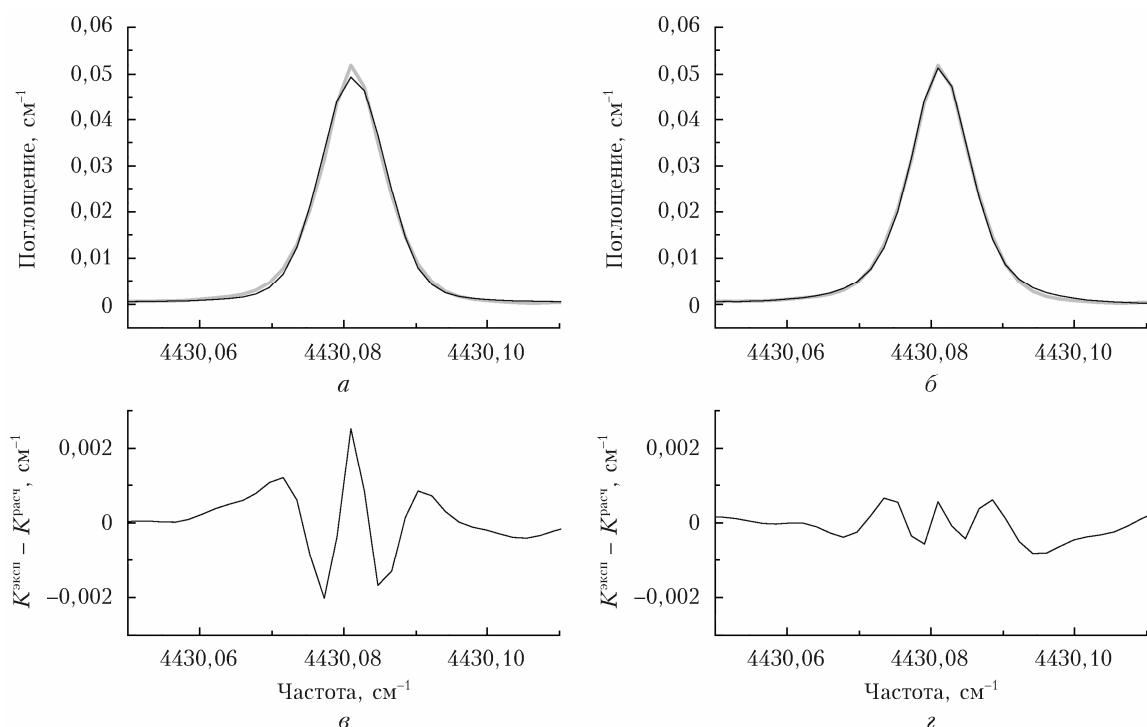
Рис. 1. Экспериментальные контуры линии 4430\text{ см}^{-1} при давлении воздуха 0 и 83 мбар, обработанные с использованием контуров V (a) и SDV (б); отклонения экспериментального контура от рассчитанного (в, г)
