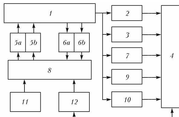
Рис. 1. Функциональная схема ОЭС обзора космического пространства
