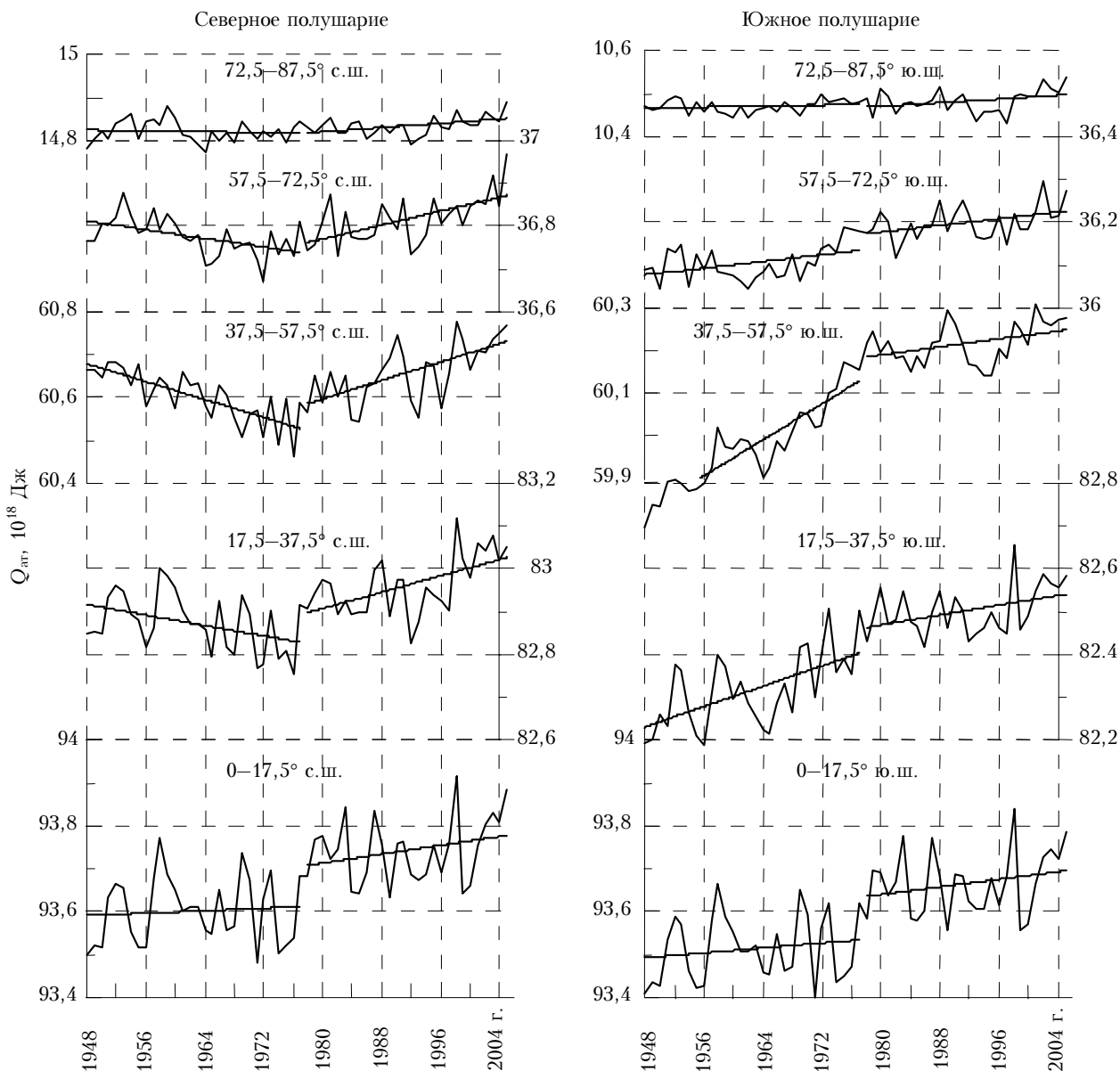
Рис. 3. Изменение теплосодержания атмосферы в слое 887–450 гПа за период 1948–2006 гг. в различных широтных зонах Северного и Южного полушарий
