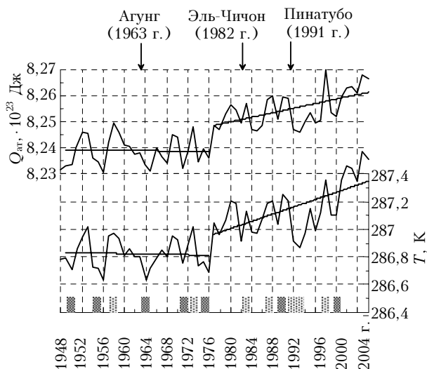
Рис. 4. Долговременные изменения теплосодержания атмосферы в слое 850–300 гПа (вверху) и приземной температуры воздуха (внизу) для всего земного шара. Стрелками указано время извержения наиболее мощных вулканов; внизу светлыми прямоугольниками – время действия Эль-Ниньо, темными – Ла-Нинья. Линии тренда проведены для периодов 1948–1977 и 1978–2006 гг.
