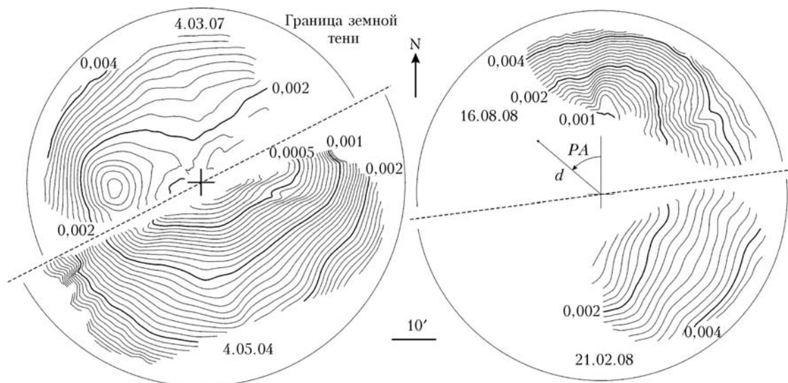
Рис. 1. Распределение величины потемнения внутри земной тени во время затмений в 2004–2008 гг. Стрелка указывает на Северный полюс мира
