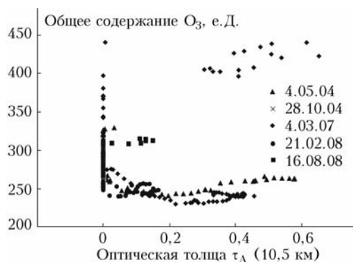
Рис. 3. Соотношение оптической толщи атмосферного аэрозоля вдоль касательной траектории с высотой перигея 10,5 км и общего содержания озона в точках лимба Земли во время лунных затмений 2004–2008 гг.
