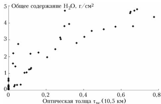
Рис. 4. Соотношение оптической толщи водяного пара вдоль касательной траектории с высотой перигея 10,5 км и общего содержания водяного пара (по данным миссии SCIAMACHY) в точках лимба Земли во время лунного затмения 4 марта 2007 г.
