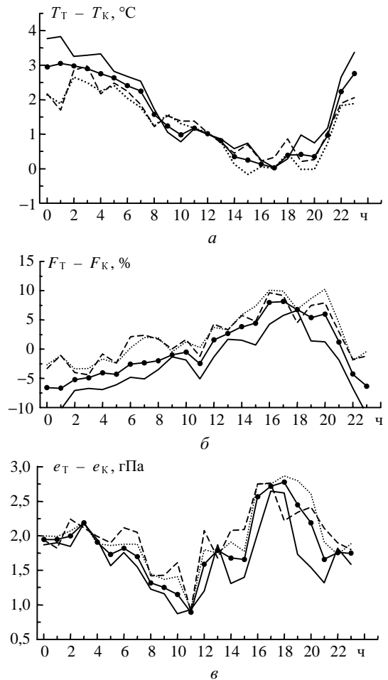
Рис. 2. Средний суточный ход разностей: a – температуры; b – относительной влажности; v – упругости водяного пара при различных направлениях ветра; ●—●—●— без учета направления ветра; ..... — с западной составляющей; ————— — с восточной составляющей; - - - - - с юго-западной составляющей
