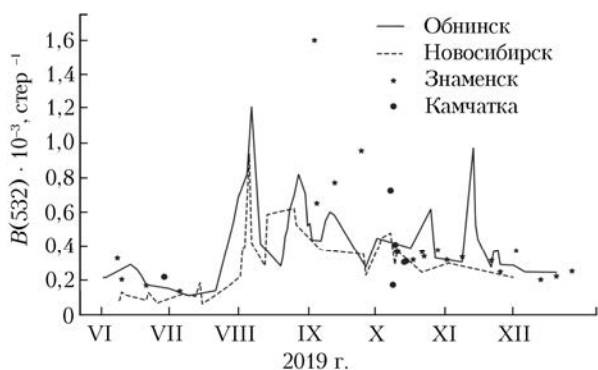
Рис. 4. Временной ход интегрального коэффициента обратного рассеяния B(532) в слое 13–18 км в июне–декабре 2019 г. на четырех станциях лидарной сети Росгидромета
