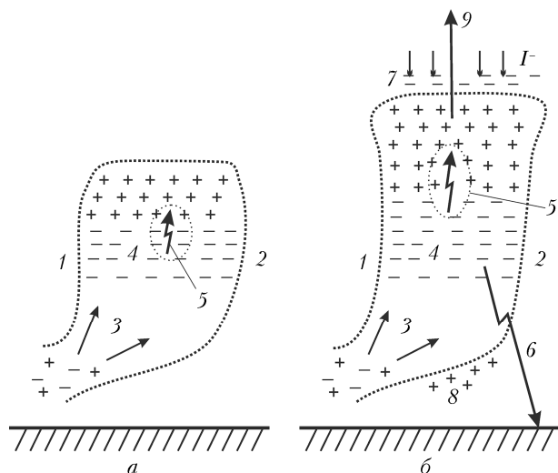
Рис. 4. Стадии образования (а) и зрелости (б) грозового облака: 1 — область теплового фронта; 2 — область холодного фронта; 3 — восходящие потоки влажного и ионизованного воздуха; 4 — область максимума частиц, создаваемых гигантским воздушным ливнем; 5 — внутриоблачная молния; 6 — молния; 7 — экранирующий слой отрицательных ионов; 8 — положительный заряд у основания облака; 9 — транзиент; I^- — ток отрицательных ионов, текущий из ионосферы к вершине облака (адаптировано из [9])
