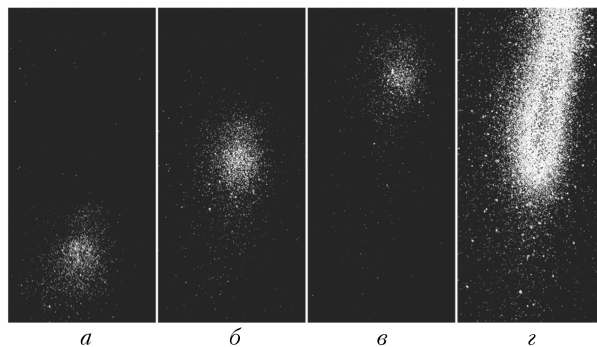
Рис. 2. Динамика апокампа при экспозиции 3 нс с интервалом 37 нс между кадрами (a–e); интегральное изображение при экспозиции 100 нс (z)
